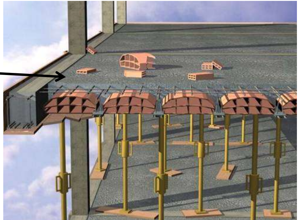
Encofrado
