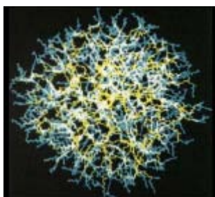
Ilustración 35. Dendrímero
