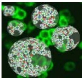
Ilustración 38. Nanopartícula
