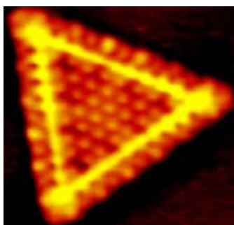
Ilustración 37. Nanocristal
