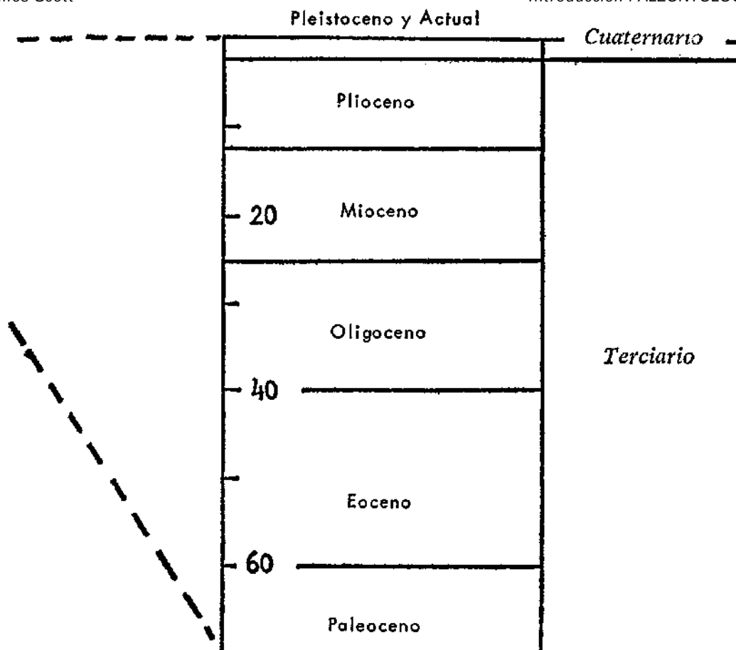
Figura 2. — La escala geológica en millones de años, con sus principales divisiones estratigráficas.
