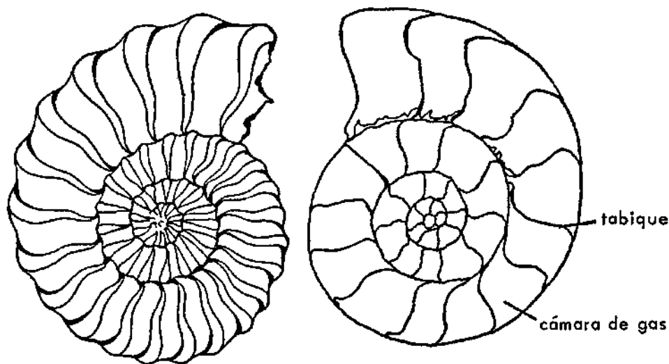
Figura 18. — Estructura de los Ammonites: a la izquierda, exterior de la concha; a la derecha, en sección sagital.
