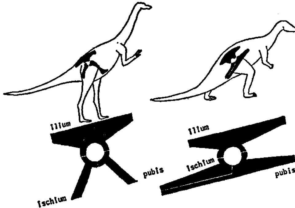
Figura 28. — Estructura de la pelvis en los Dinosaurios, en relación con su clasificación en Saurisquios (izquierda) y Ornitisquios (derecha).
