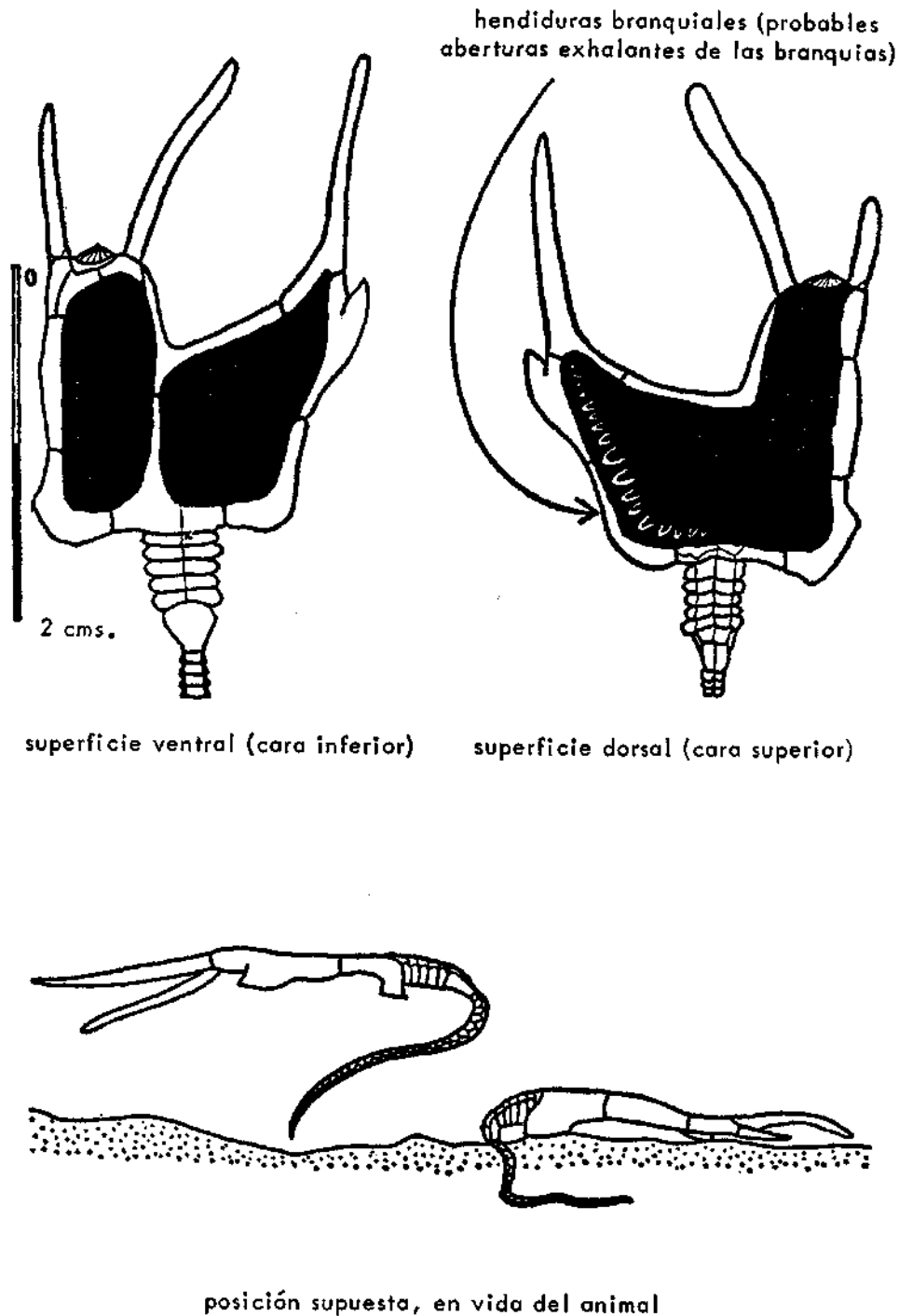
Figura 14. — Estructura de Cothurnocystis , un representante de los Calcicordados.
