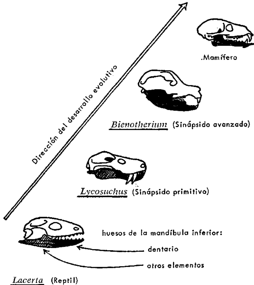
Figura 5. — Evolución de la mandíbula en el tránsito de Reptil a Mamífero (los dibujos no están a escala).
