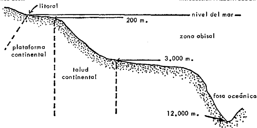
Figura 15. — Regiones faunísticas consideradas en el mar.
