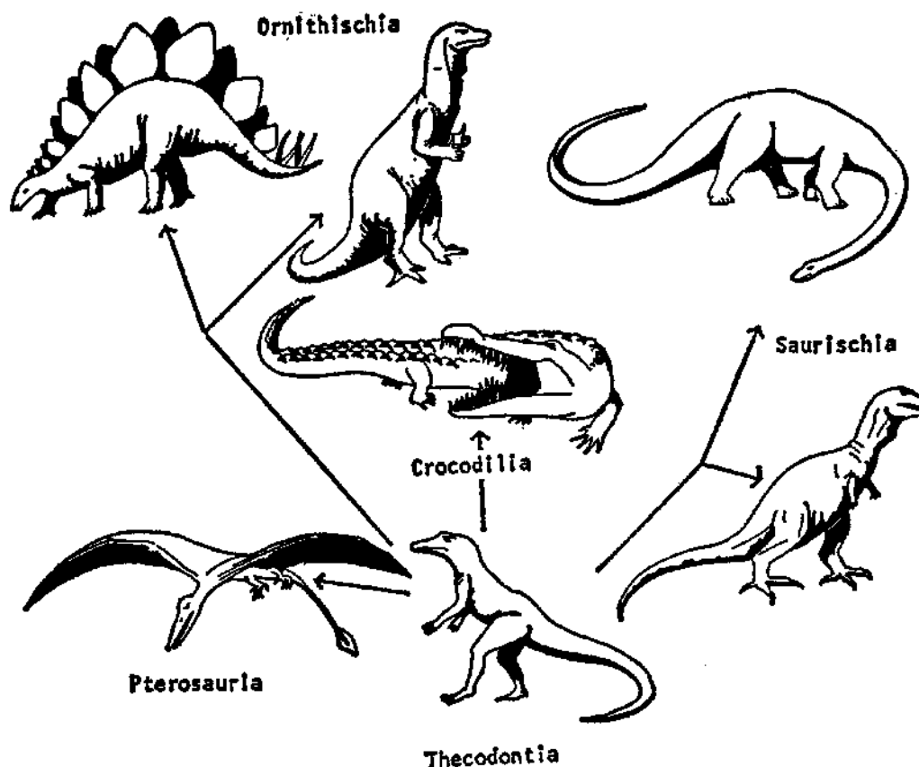
Figura 29 — Evolución y radiación de los Arqueosaurios. (Los dibujos no están hechos a escala,)
