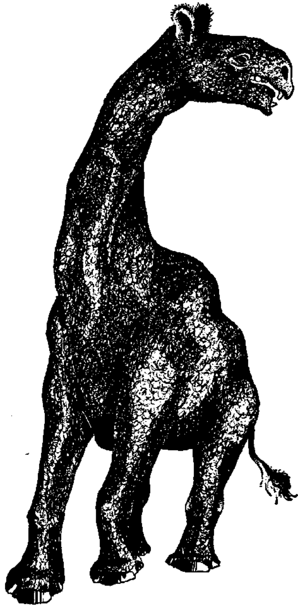
Figura. 31. — Indricotherium , un Mamífero ungulado, gigantesco, del Oligoceno, de 6 m. de alzada.
