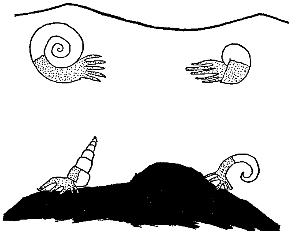
Figura 19. — Posición biológica supuesta para diversos Ammonoideos vivos. Los Ammonites de la parte superior, de conchas normales, nadan libremente. Los dos de la parte inferior, «heteromórficos», corresponden a los géneros Turrilites (izquierda), y Crioceras (derecha); ambos debían ser bentónicos.
